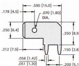
.250 (6.4) TAB
