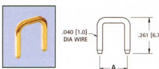
.040 (1.0) PINS
