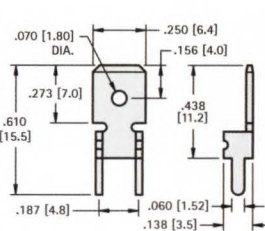
.250 (6.4) TAB
