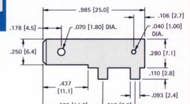
.250 (6.4) TAB
