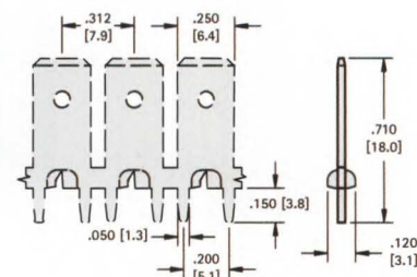
.250 (6.4) TAB
