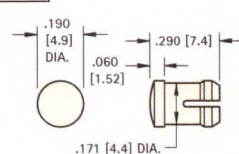
FIG. 3 T-1
