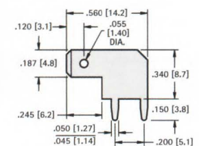
.187 (4.8) TAB
