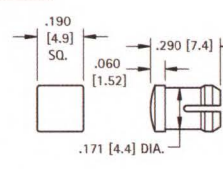
FIG. 6 T-1
