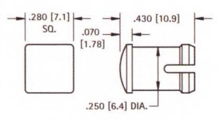
FIG. 7 T-1 3/4
