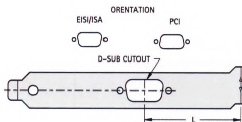
D-SUB
