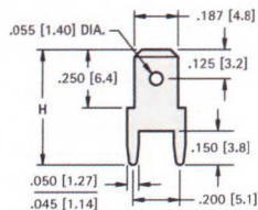
.187 (4.8) TAB
