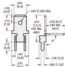
.250 (6.4) TAB
