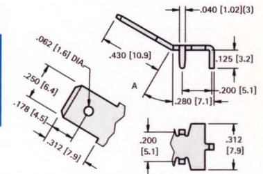
.250 (6.4) TAB
