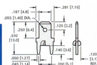
.187 (4.8) TAB
