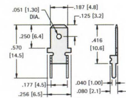
.187 (4.8) TAB
